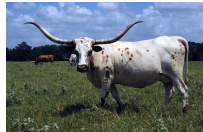
LLL SPECKLES
